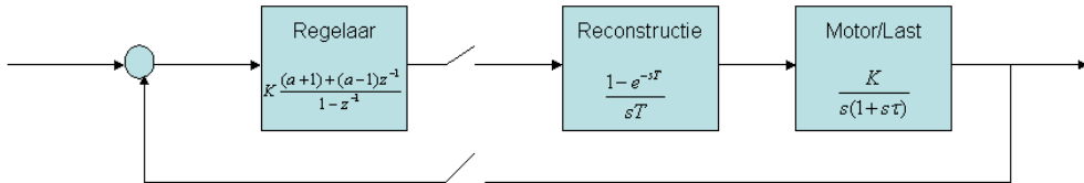
Fig. 1: Voorbeeld van een servo met digitale PI regelaar, de schakelaars stellen de bemonstering voor. Het reconstructiefilter is een nulde-orde extrapolator (de waarde op het bemonsteringsmoment wordt vastgehouden tot het volgende (sample&hold)).
