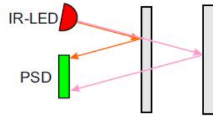
GP2D12
